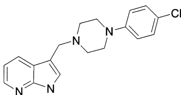
L-745,870
